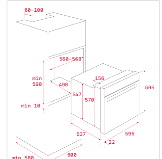
HLB 860 - HLB 8400 - HLB 850 - HLB 840 HLB 830 - HSB 645 - HSB 640 - HSB 635 HSB 630 - HSB 615 - HSB 610 - HCB 6535 HCB 6525 - HRB 6300 - HRB 6100 - HBB 605 HBB 535 - HBB 510 - HBB 435 - HBB 490
