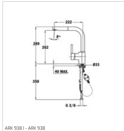
ARK 938 I - ARK 938
