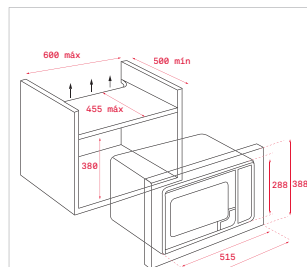
VS 152 GS - CP 15 GS - VS 1520 GS CP 150 GS
